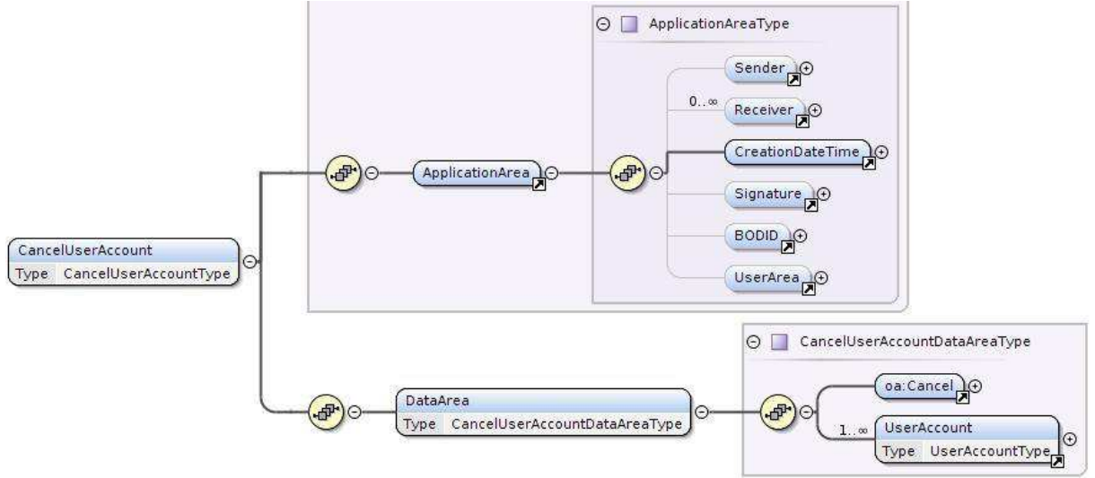
Şekil 7 Kullanıcı İptal/Silme Mesaj Yapısı
